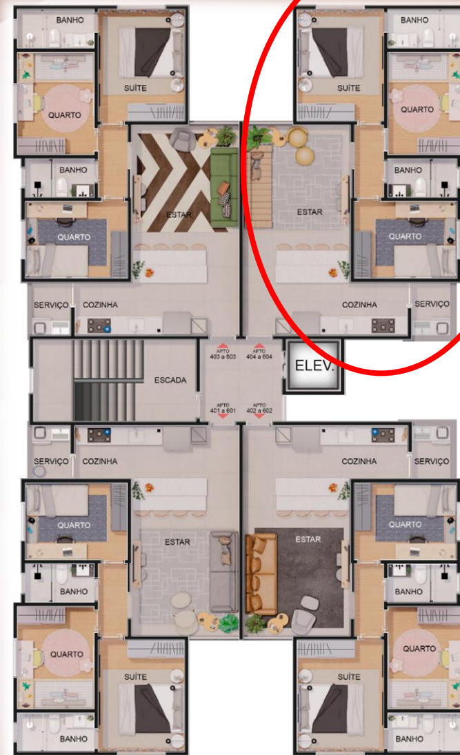
PLANTA 4º a 6º PAVIMENTO - APARTAMENTOS TIPO
